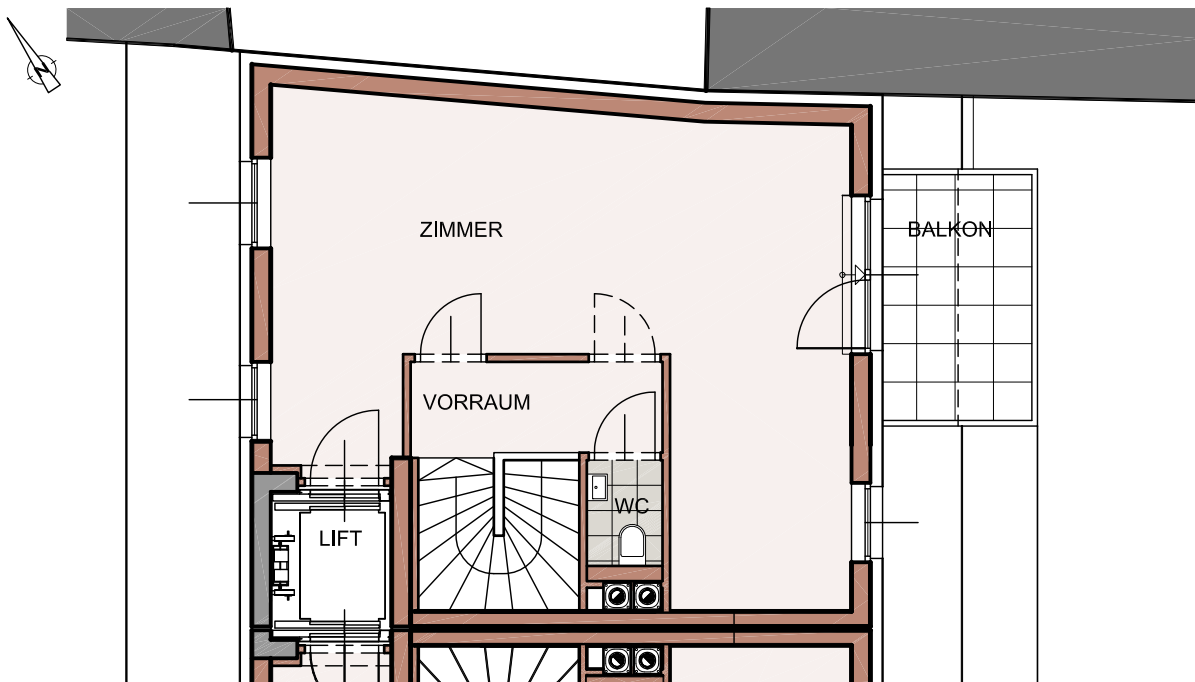
GRUNDRISS OG2 VARIANTE OHNE TEILUNG M 1:100
