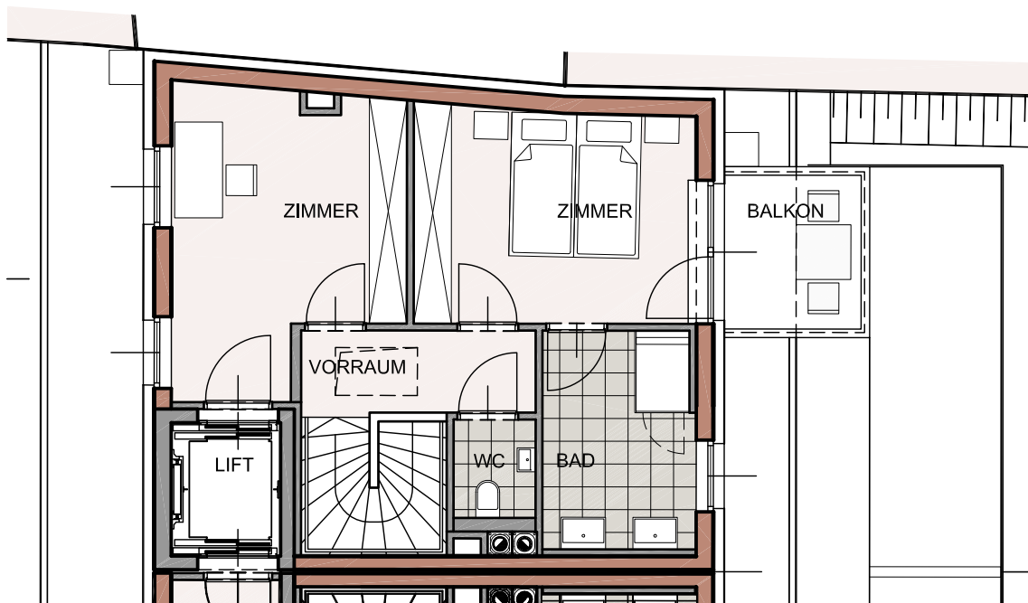
GRUNDRISS OG2 VARIANTE MIT TEILUNG M 1:100
