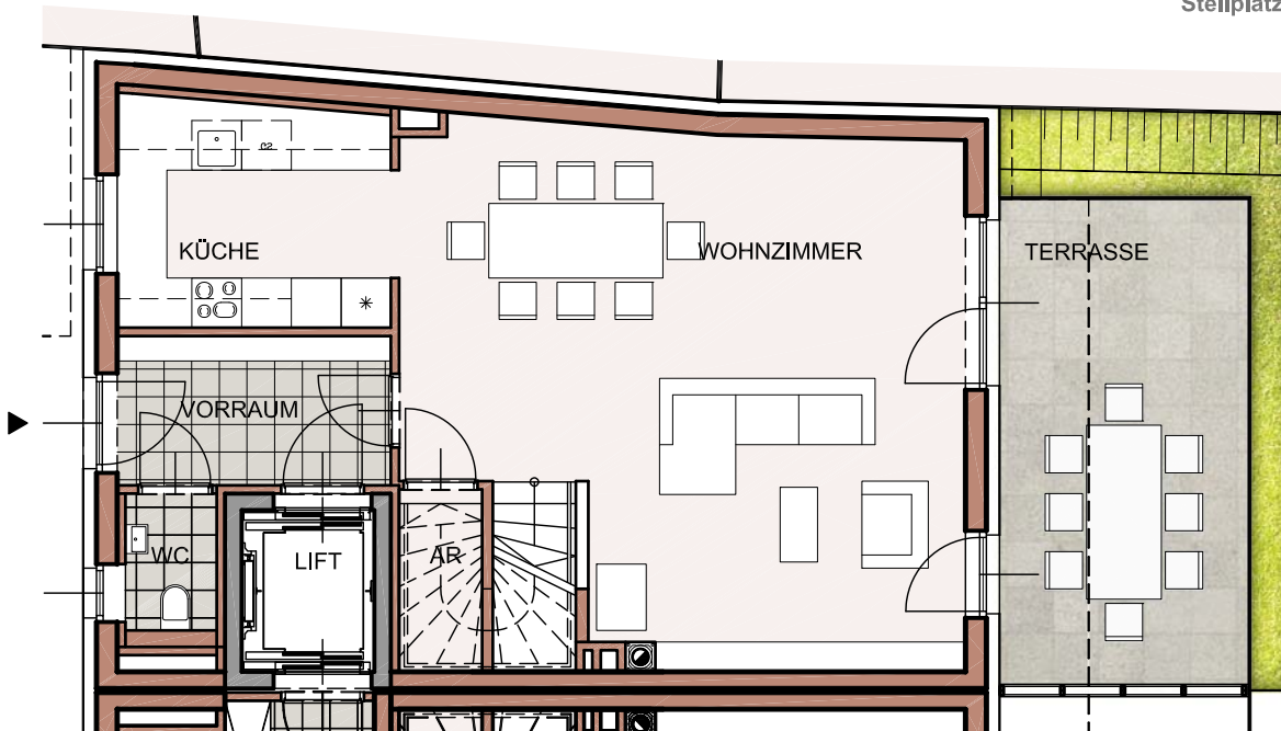
GRUNDRISS EG M 1:100
